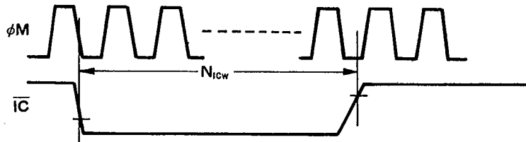
Fig. A-2 Reset Timing
